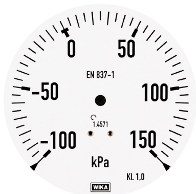
enkelgraderad skala kPa
