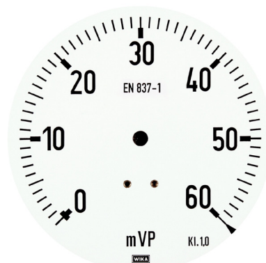
enkelgraderad skala mvp
