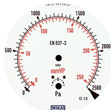
dubbelgraderad skala mmvp/Pa
