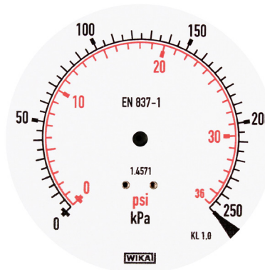
dubbelgraderad skala psi/kPa
