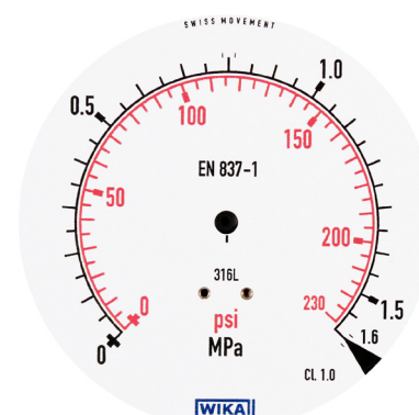
dubbelgraderad skala psi/MPa
