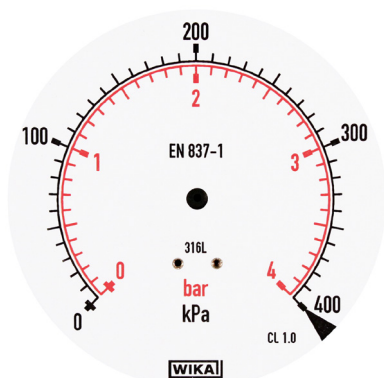
dubbelgraderad skala bar/kPa
