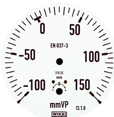
enkelgraderad skala mmvp
