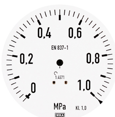
enkelgraderad skala MPa
