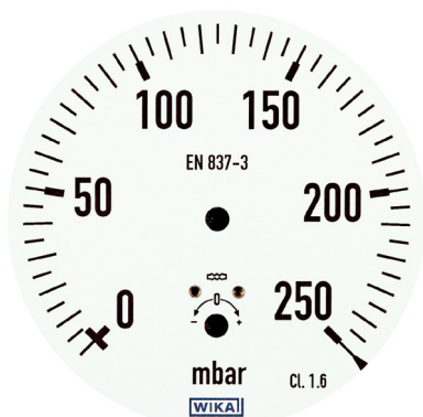
enkelgraderad skala mbar
